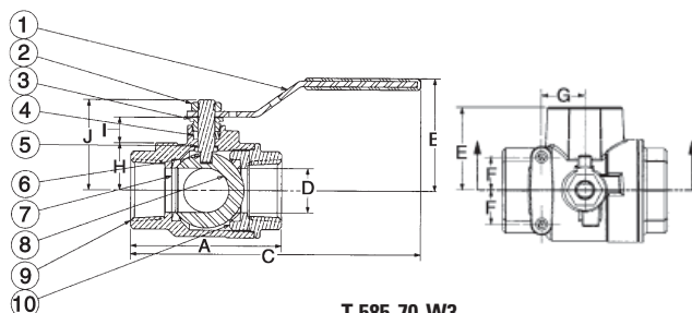
T-585-70-W3
