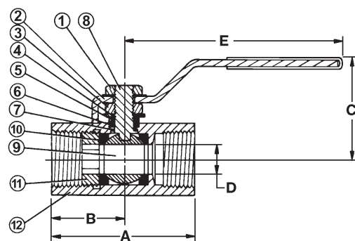
T-570-CS-R-25
