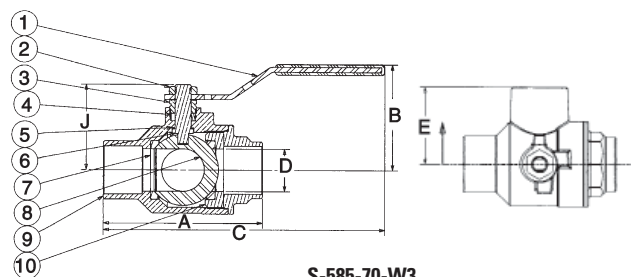
S-585-70-W3
