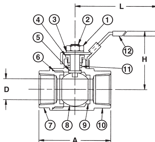
TC-580-CS-R-66-LL
