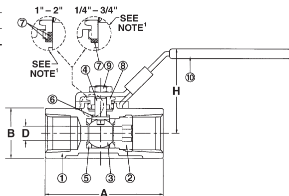
T-560-CS-R-66-LL
